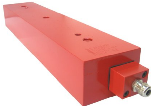
Electroimants rectangulars amb sortida de cable en diferents posicions.
